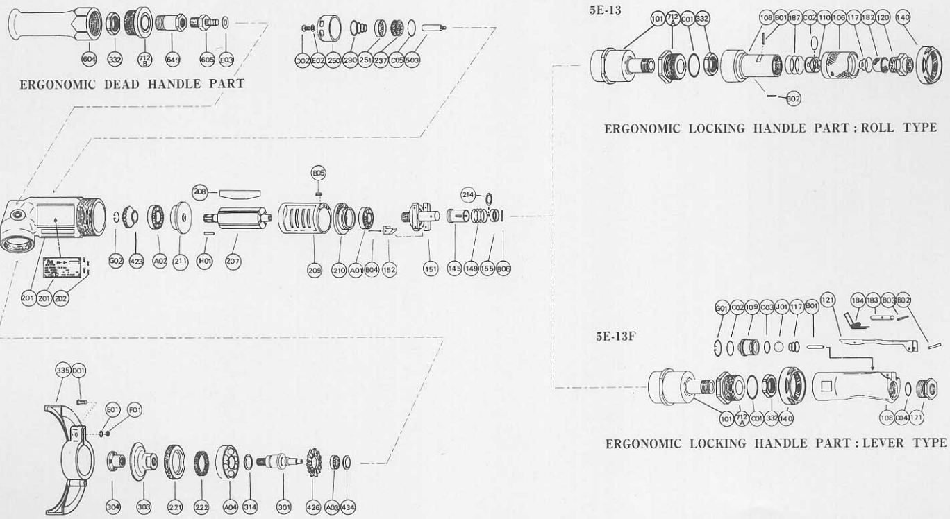
FA-5E-13, -13F
